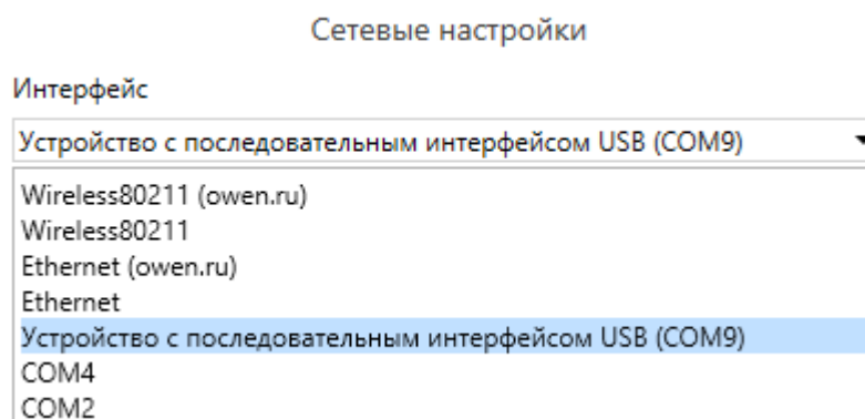
Рисунок 7.2 – Выбор интерфейса
